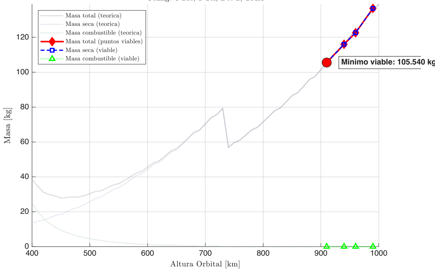
Desglose de Masas vs. Altura Config: 3 Sat, 1 Tel, Det 2, TMA
